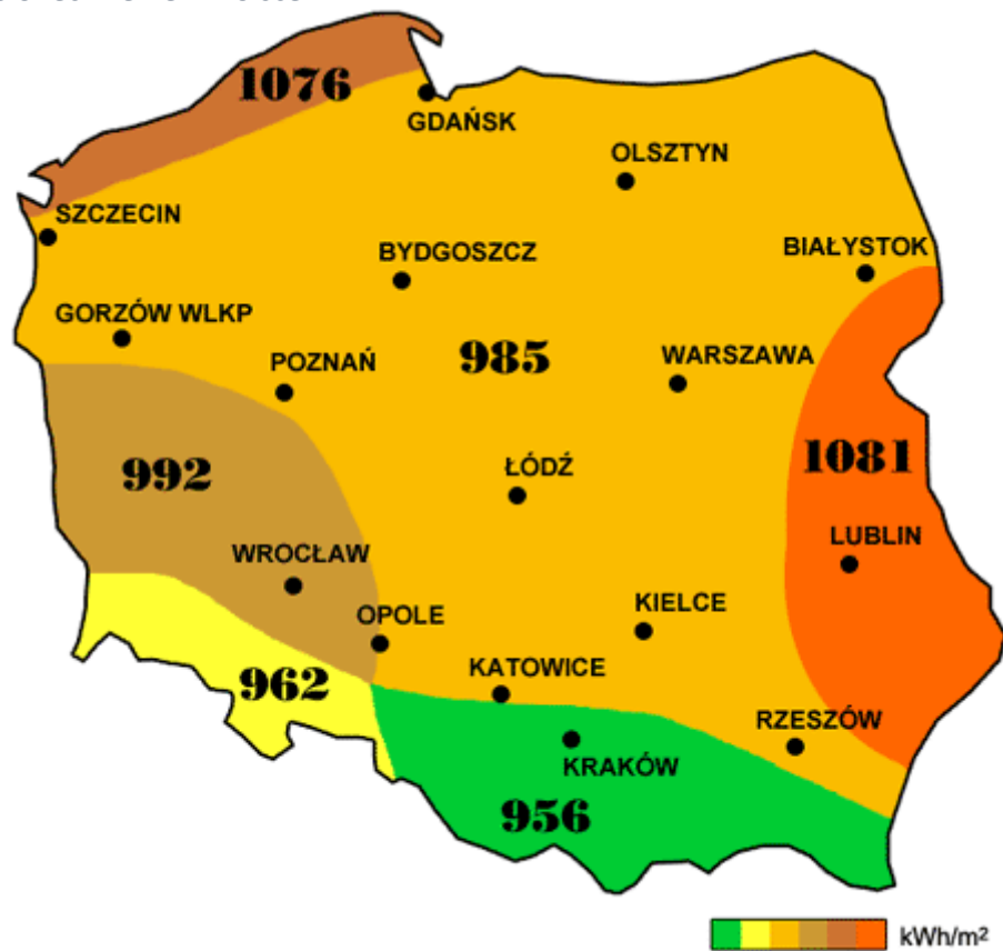
Mapa 6. Nasłonecznienie w Polsce
